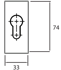
Square Escutcheon
